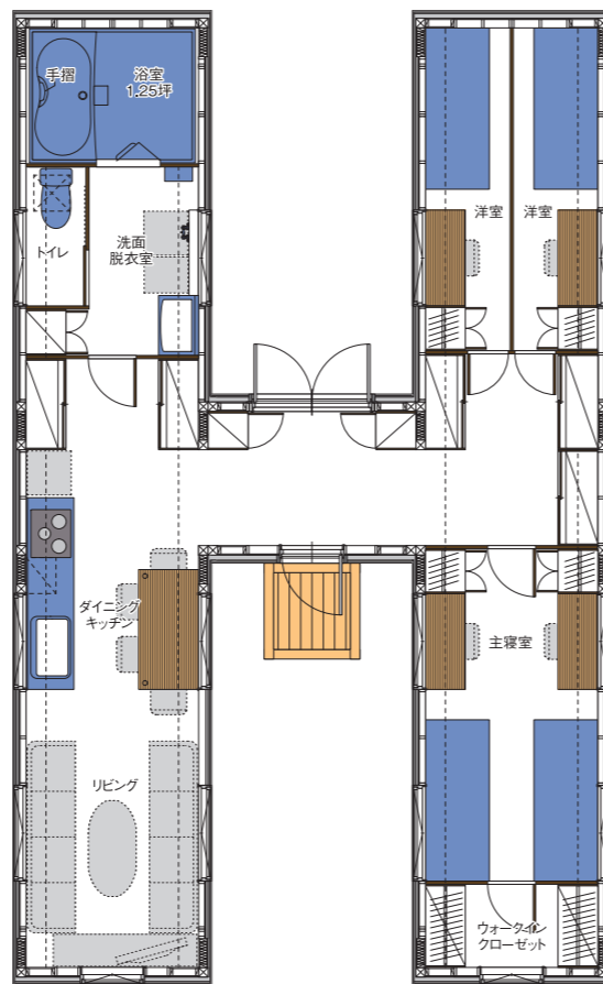
住居棟 (4P)
