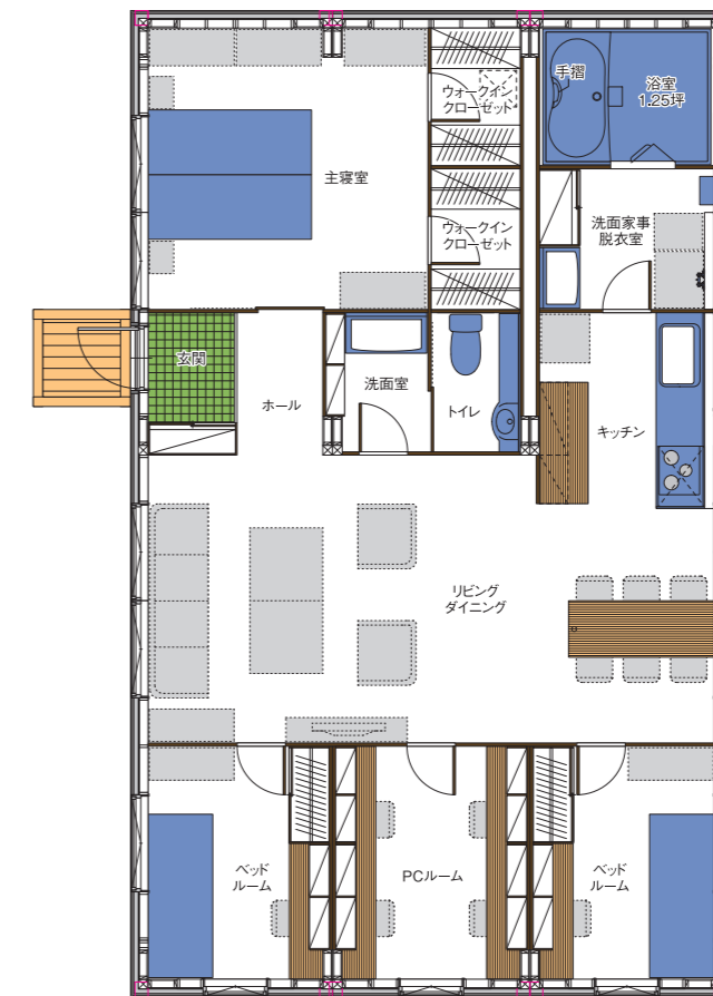
住居棟 (4P)
