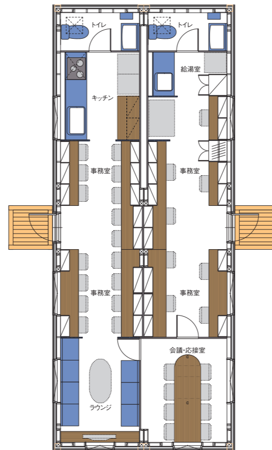
食堂・事務・ラウンジ棟 (24P)
